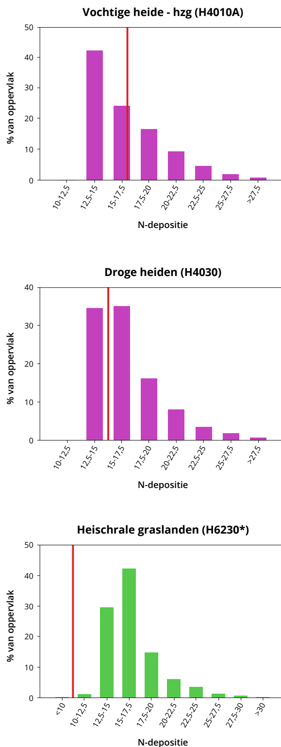
Figuur 4.9. Verdeling van de stikstofdepositie per 2,5 kg N/ha/jaar-klasse voor vochtige heide (hogere zandgronden) (H4010A), droge heide (H4030) en heischrale graslanden (H6230*) als percentage van het totaal oppervlak. De rode lijn geeft de KDW van het type weer.
