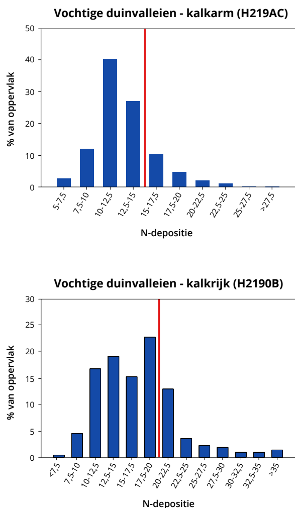
Figuur 4.2. Verdeling van de stikstofdepositie per 2,5 kg N/ha/jaar-klasse voor het habitatype vochtige duinvalleien (H2190AC & H2190B) als % van het totaal oppervlak. De rode lijn geeft de KDW weer. Voor H2190AC is de KDW 14 of 15 kg N/ha/jaar. 2,5 kg N/ha/jaar komt overeen met 178 mol N/ha/jaar.
