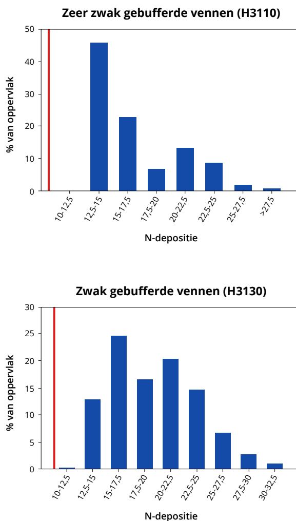
Figuur 4.8. Verdeling van de stikstofdepositie per 2,5 kg N/ha/jaar-klasse voor zeer zwak gebufferde vennen (H3110) en zwak gebufferde vennen (H3130) als percentage van het totaal oppervlak. De rode lijn geeft de KDW van het type weer.
