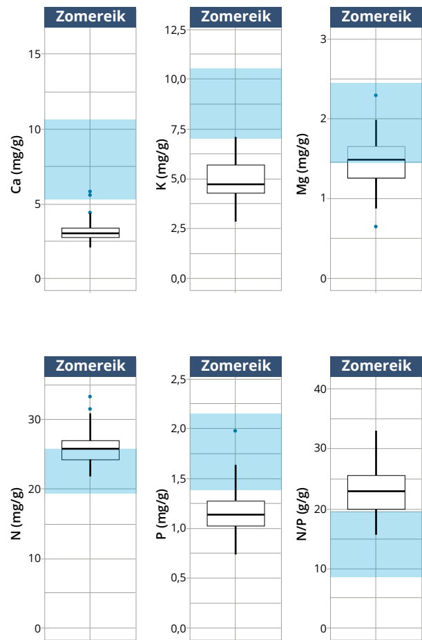
Figuur 5.12. Overzicht van de bladchemie (boxplots) van zomereik (augustus 2020, n=30 ) in oude eikenbossen op de Veluwe (naar Weijters et al. 2020). De blauwe band geeft de range van goede plantenvoeding weer voor zomereik (Mellert & Göttlein 2012).
