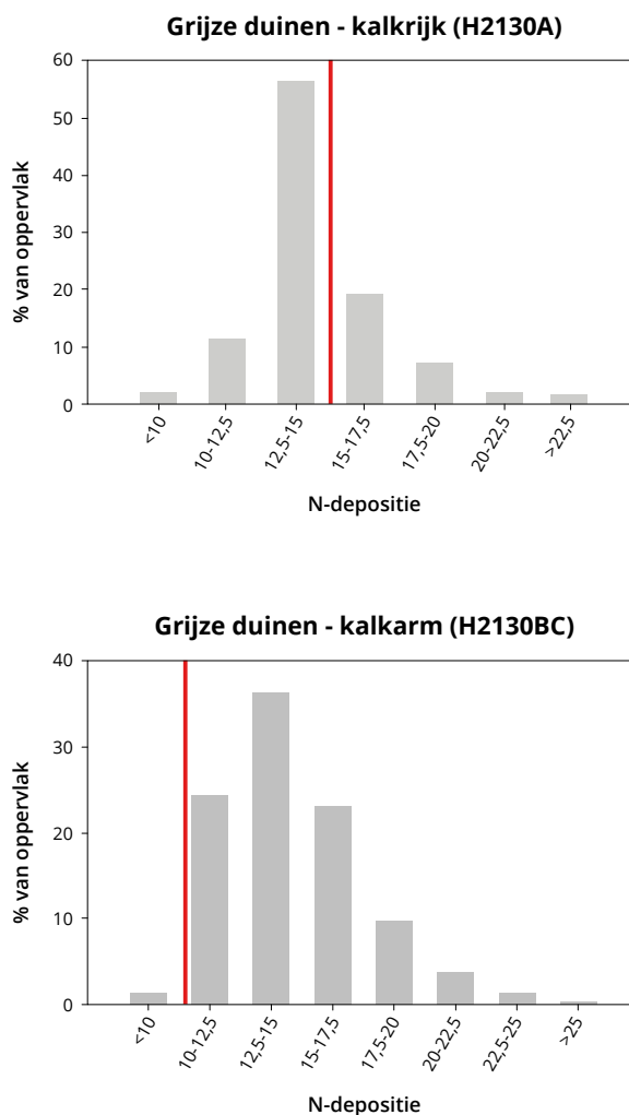
Figuur 4.1. Verdeling van de stikstofdepositie per 2,5 kg N/ha/jaar-klasse voor het habitatype Grijze duinen (H2130A & H2130BC) als percentage van het totaal oppervlak. De rode lijn geeft de KDW van het type weer. 2,5 kg N/ha/jaar komt overeen met 178 mol N/ha/jaar.
