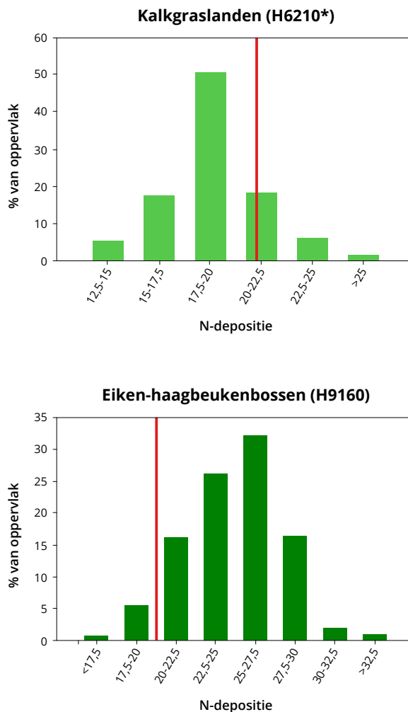
Figuur 4.12. Verdeling van de stikstofdepositie per 2,5 kg N/ha/jaar-klasse voor het habitatype kalkgraslanden (H6210) en eiken-haagbeukenbossen (H9160) als percentage van het totaal oppervlak. De rode lijn geeft de KDW van het type weer.
