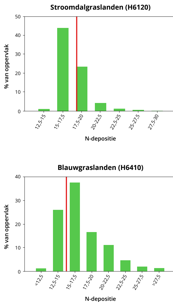
Figuur 4.6. Verdeling van de stikstofdepositie per 2,5 kg N/ha/jaar-klasse voor het habitattype stroomdalgraslanden (H6120) en blauwgraslanden (H6410) als percentage van het totaal oppervlak. De rode lijn geeft de KDW van het type weer.
