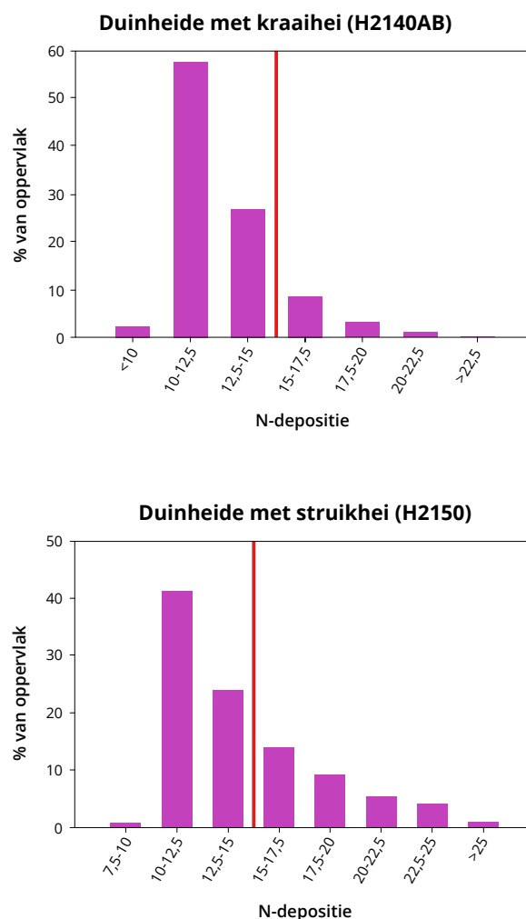
Figuur 4.3. Verdeling van de stikstofdepositie per 2,5 kg N/ha/jaar-klasse voor de habitattypen duinheide met kraaihei (H2140) en duinheide met struikhei (H2150) als percentage van het totaal oppervlak. De rode lijn geeft de KDW van het type weer.
