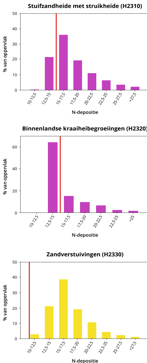
Figuur 4.7. Verdeling van de stikstofdepositie per 2,5 kg N/ha/jaar-klasse voor stuifzandheide met struikhei (H2310), binnenlandse kraaiheibegroeiingen (H2320) en zandverstuivingen (H2330) als percentage van het totaal oppervlak. De rode lijn geeft de KDW van het type weer.
