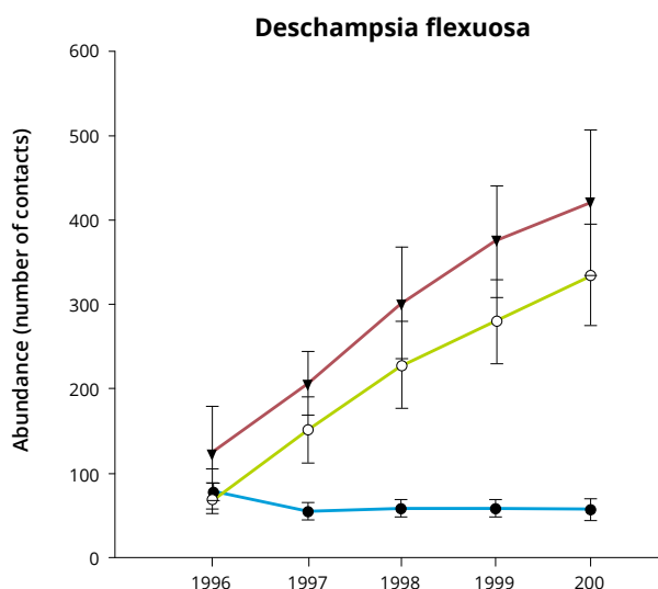
Figuur 5.3. Abundantie van het gras bochtige smele ( Deschampsia flexuosa ) bij twee niveaus van stikstoftoediening (groen: 12,5 kg N/ha/jaar & rood 50 kg N/ha/jaar) in een boreaal naaldbos in Midden Zweden (Nordin et al. 2005). De blauwe lijn is de onbehandelde controle.
