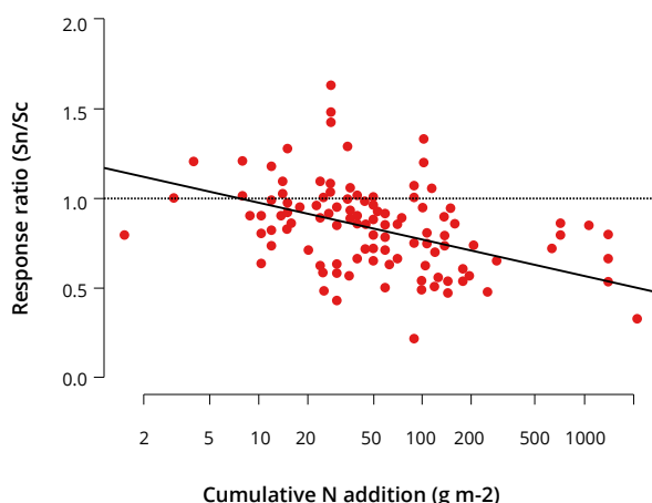
Figuur 6.4. Verband tussen de soortenrijkdom responsratio (Soortenaantal bij N-additie/Soortenaantal in controle). Is deze waarde 1, dan is er geen effect van stikstofgift, 0,5 komt overeen met 50% reductie t.o.v. de controle (Soons et al. 2017). Een stikstofbelasting van 100 g N/m² komt overeen met 1000 kg N/ha. NB.: x-as is logaritmisch uitgezet.
